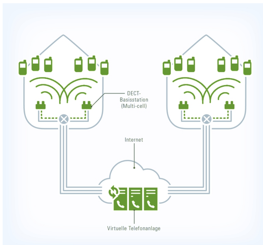
Abbildung 3: DECT-Multi-cell
