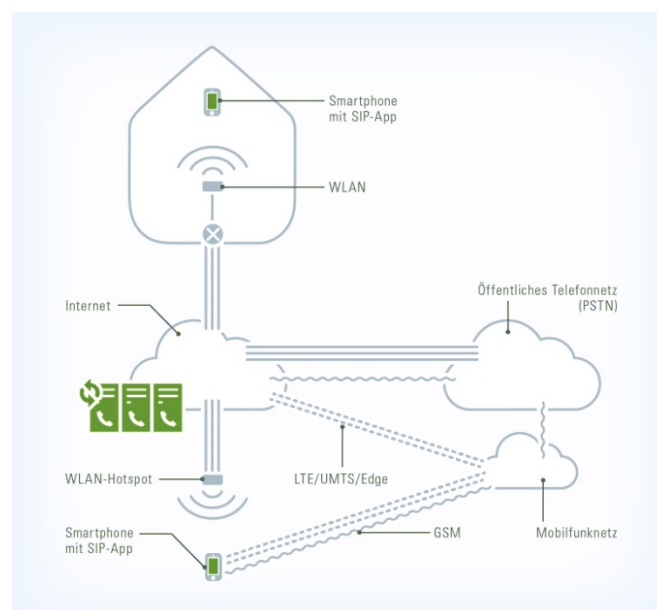
Abbildung 2: Mobilfunk Integration
